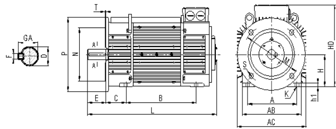
卧式、机座带底脚，端盖带凸缘
